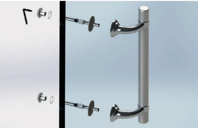
KIT 4 fissaggio coppie per porte: vetro
