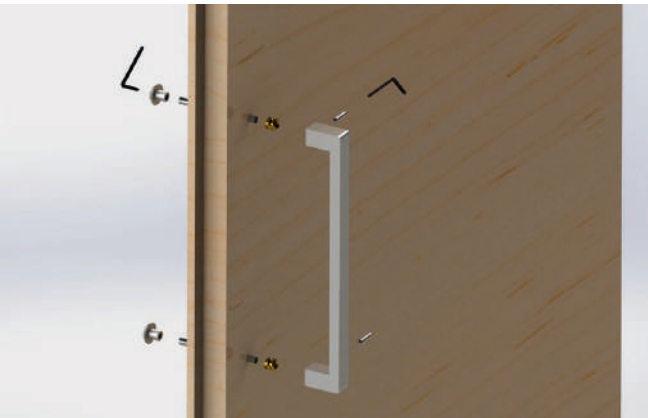
KIT 15 fissaggio maniglione singolo / inox / passante
